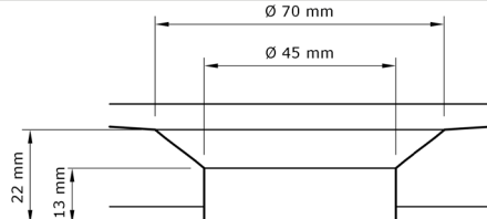
DETAGLIO ZONA SCARICO/EINZELHEIT ABFLUSS
